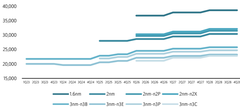
圖表 4：晶圓價格趨勢
